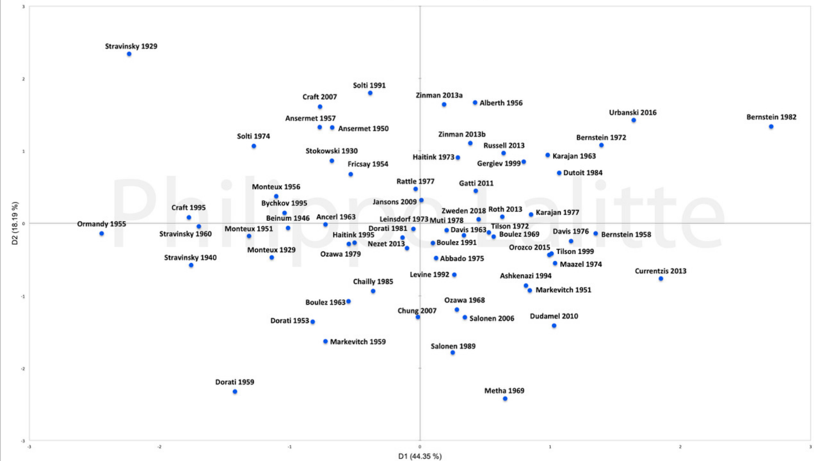
Observations (axes D1 et D2 : 62.54 %)
